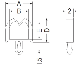
P.C.B Ø1.75 THICKNESS 1.6
