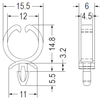
CHASSIS: ØG THICKNESS 0.8-2.2
