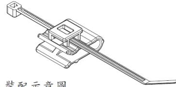
装配示意图
