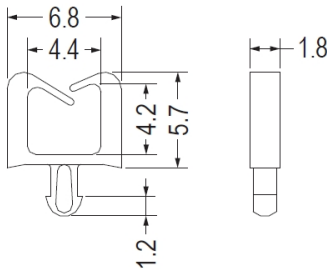
P.C.B Ø1.75 THICKNESS 1.6
