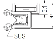
装配示意图
